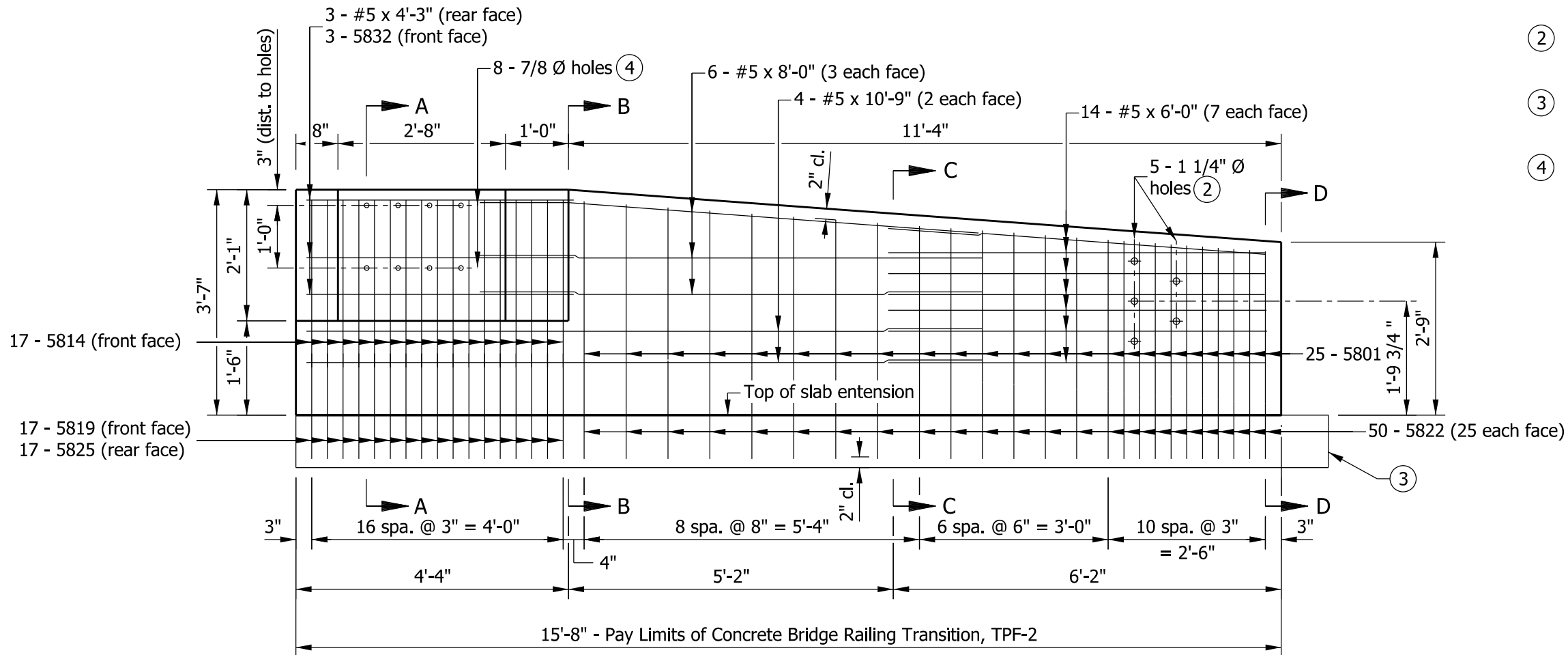
ELEVATION
