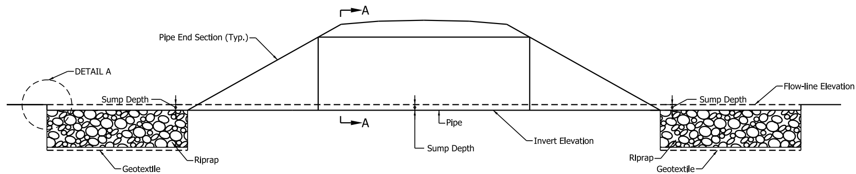
ELEVATION
