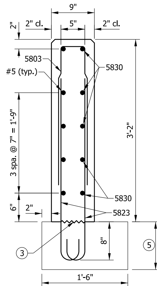
SECTION D-D
