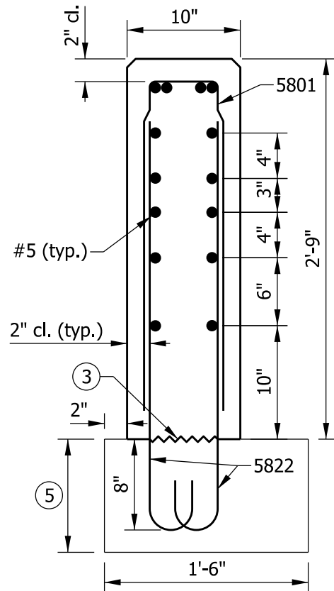
SECTION D-D
